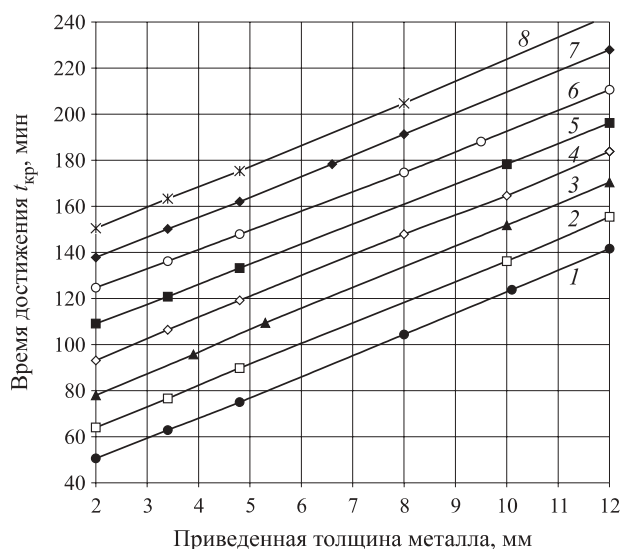
Рис. 5. Огнестойкость стальных конструкций с огнезащитной облицовкой из плит PYRO-SAFE AESTUVER T при t_{кр} = 550 °C при их толщине: 1 — 15 мм; 2 — 20 мм; 3 — 25 мм; 4 — 30 мм; 5 — 35 мм; 6 — 40 мм; 7 — 45 мм; 8 — 50 мм
