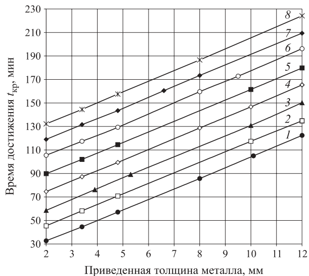
Рис. 3. Огнестойкость стальных конструкций с огнезащитной облицовкой из плит PYRO-SAFE AESTUVER T при t_{кр} = 450 °С при их толщине: 1 — 15 мм; 2 — 20 мм; 3 — 25 мм; 4 — 30 мм; 5 — 35 мм; 6 — 40 мм; 7 — 45 мм; 8 — 50 мм
