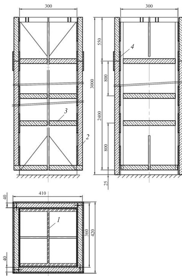
Рис. 1. Пример конструктивной схемы огнезащитной облицовки из плит PYRO-SAFE AESTUVER T плотностью 650 \text{ кг/м}^3 \pm 10 \% : 1 — двутавровая балка; 2 — огнезащитные плиты PYRO-SAFE AESTUVER T толщиной 40 мм; 3 — ребра жесткости из плит толщиной 40 мм, с выступом на 10 мм от полок двутавра; 4 — пояса шириной (100±10) мм из плит PYRO-SAFE AESTUVER T толщиной 10 мм
