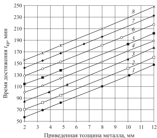
Рис. 6. Огнестойкость стальных конструкций с огнезащитной облицовкой из плит PYRO-SAFE AESTUVER T при t_{кр} = 600 °C при их толщине: 1 — 15 мм; 2 — 20 мм; 3 — 25 мм; 4 — 30 мм; 5 — 35 мм; 6 — 40 мм; 7 — 45 мм; 8 — 50 мм
